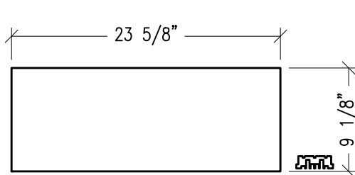
TOP
