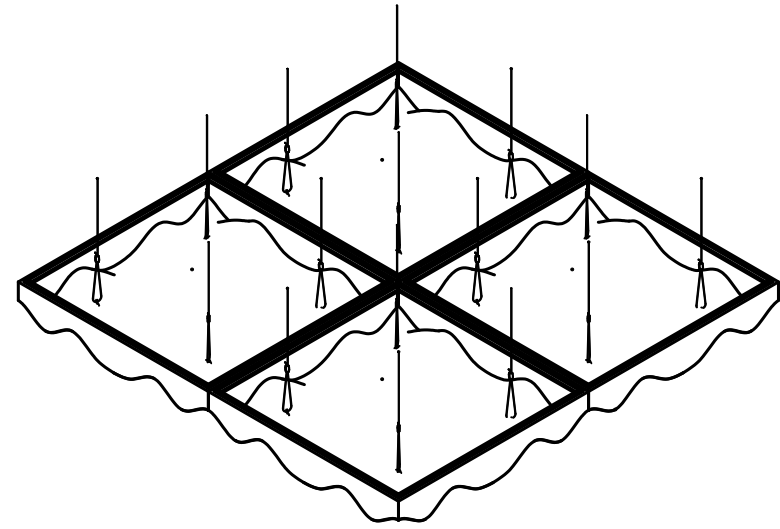
BICUBIC ARRAY
