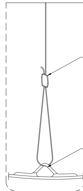
HANGROD DETAIL
