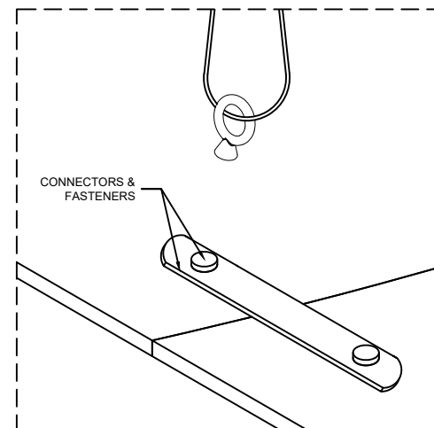
D1 DETAIL SCALE: NONE ARCH'T REF.:
