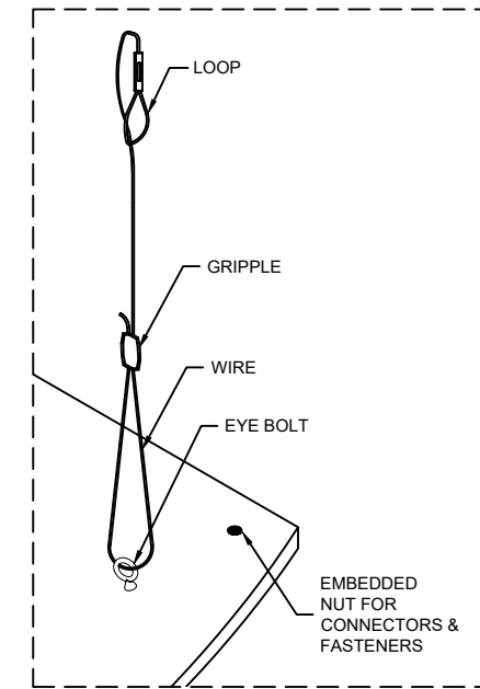
D1 DETAIL SCALE: NONE ARCH'T REF.:
